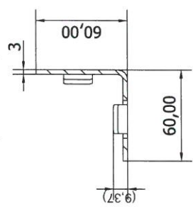
A-A (0,40:1)
