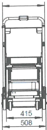
Schemat wymiarów
