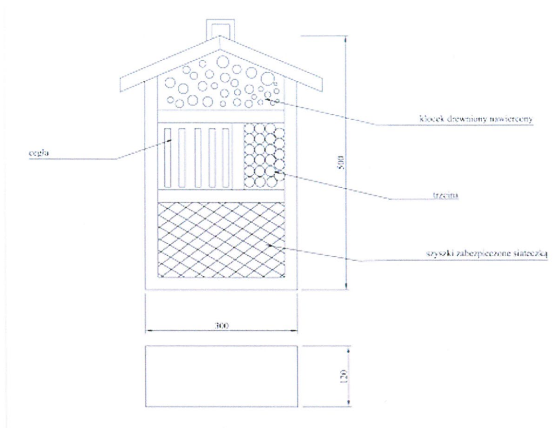
Rysunek techniczny domku dla owadów
